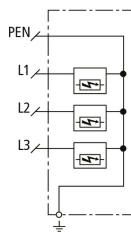
Prinzipschaltbild DSH ZP 2 TNC 255
