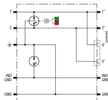
Principalschaltbild DBX TC B 180
