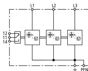
Prinzipialschaltbild DSH B TNC 255 FM
