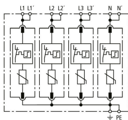
Prinzip Schaltbild DG MP TNS 275
