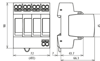
Maßbild DG MP TNS 275
