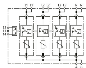
Prinzipialschaltbild DG MP TNS 275 FM
