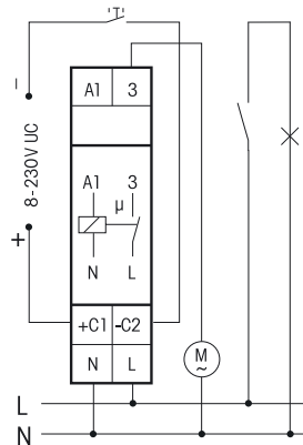
Ventilatorsteuerung über Kleinspannungs-Türkontakt, Licht getrennt geschaltet
