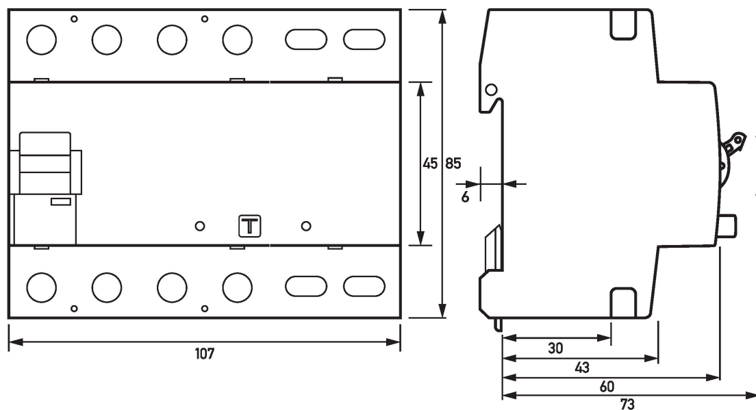
Maßzeichnung DFS 6 A NU, 4-polig (Gruppenansicht)
