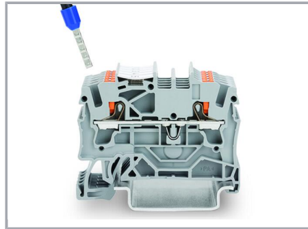
Direktes Stecken (Push-in) – eindrätige Leiter und Leiter mit Aderendhülse
