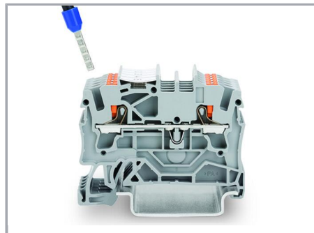
Direktes Stecken (Push-in) – eindrängige Leiter und Leiter mit Aderendhülse
