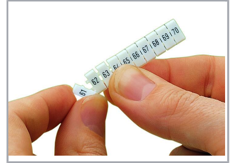
Trennen eines Einzelschildchens vom WMB-Beschriftungsstreifen, für größere Klemmenbreiten
